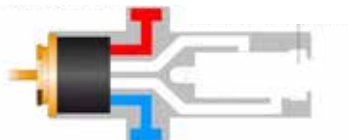
Thermostatische mengkraan zonder keerkleppen Service van de therm. patroon mogelijk, in gesloten stand. Zonder het water af te sluiten!
