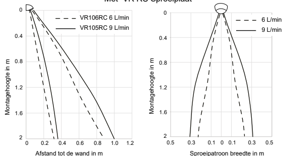
Sproei patronen Met "VR RC Sproeiplate"
